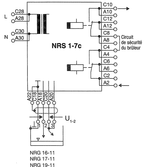
Schéma de raccordement du commutateur de niveau type NRS 1-7c/d
