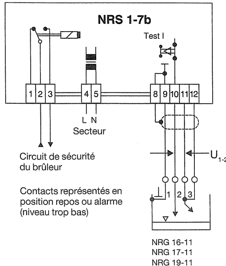
Schéma de raccordement du commutateur de niveau type NRS 1-7b
