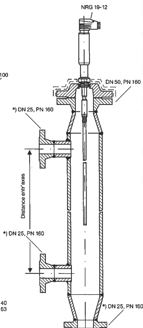
Fig. 5: Bouteille extérieure (bouteille de mesure type III) pour l'installation de l'électrode
