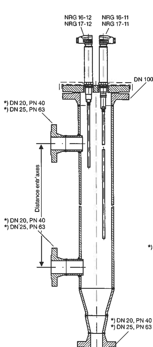
Fig. 4: Bouteille extérieure (bouteille de mesure type XIII) pour l'installation des électrodes
